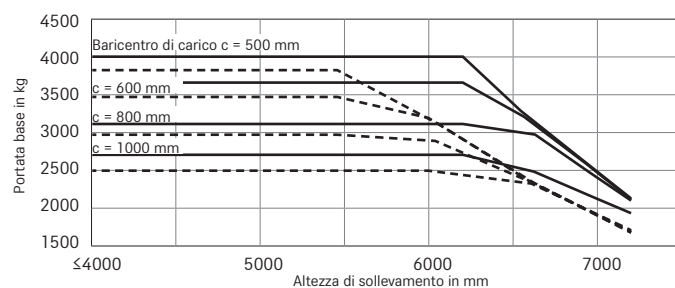
RX 70-40 Montante triplex Gommatura superelastica semplice
