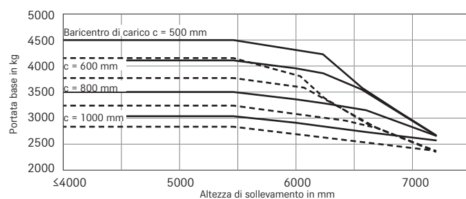
RX 70-45 Montante triplex Gommatura superelastica semplice
