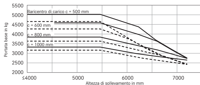
RX 70-50 Montante triplex Gommatura superelastica semplice
